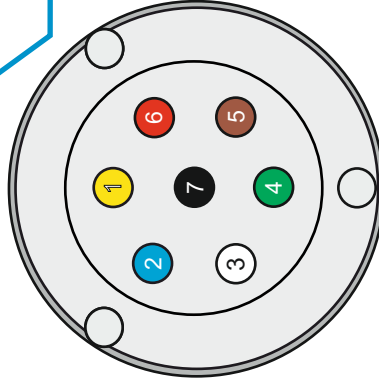
Вид розетки со стороны подключения проводов ISO1724
